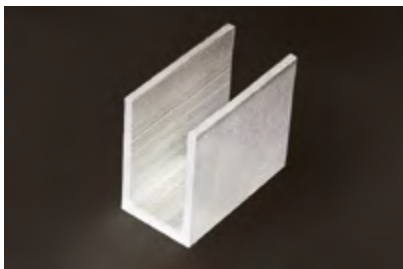
Soporte U 80x40 Aluminio
